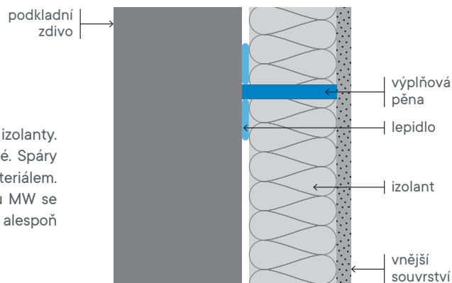
Schéma výplně spáry
