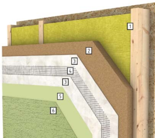
Obr. 1: Schéma skladby omítkového systému a podkladu
